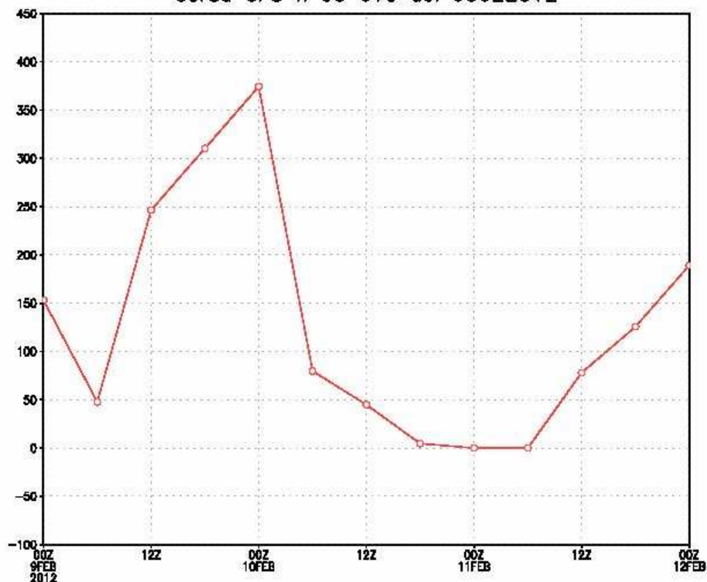
altezza zero termico su Ancona corsa GFS h 00 UTC del 08022012
