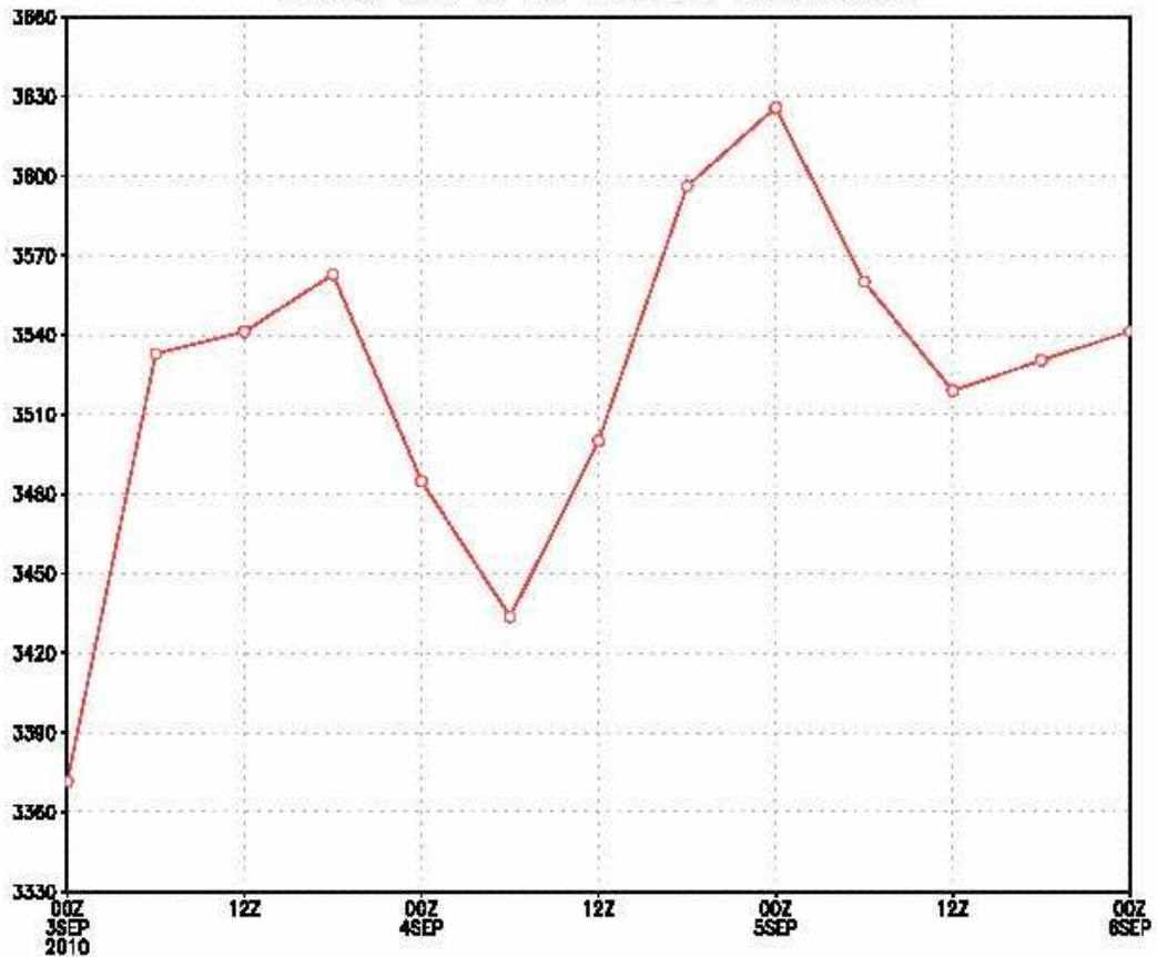
altezza zero termico su Ancona corsa GFS h 00 UTC del 02092010
