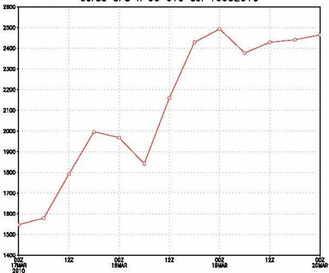
altezza zero termico su Ancona corsa GFS h 00 UTC del 16032010
